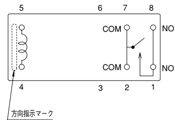
●端子配列・内部結線図 (BOTTOM VIEW)
