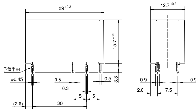
●外形寸法図 FTR-K1CK( ) W-HT 形
