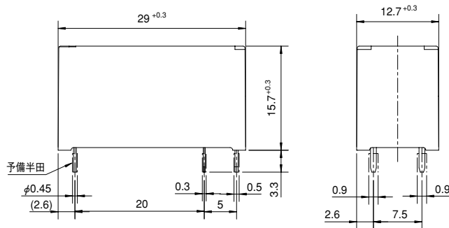
●外形寸法図 FTR-K1AK( ) T-HT 形
