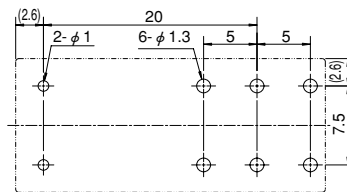
●プリント基板加工図 (BOTTOM VIEW)
