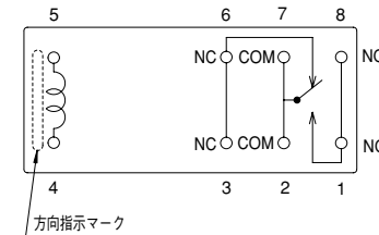
●端子配列・内部結線図 (BOTTOM VIEW)
