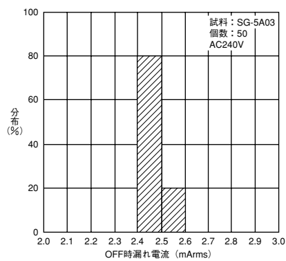
OFF時漏れ電流の分布
